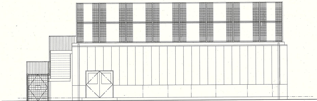
倉庫棟 南側立面図
