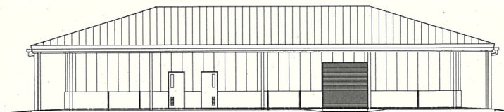
クラブハウス棟 北側立面図
