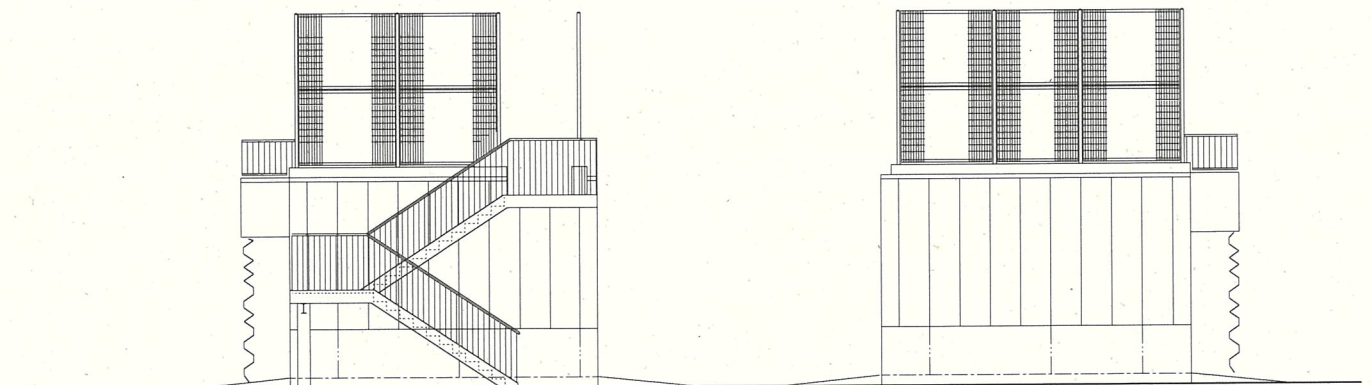
倉庫棟 西側立面図
