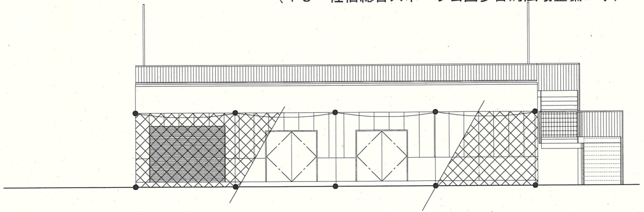
倉庫棟 北側立面図
