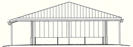
クラブハウス棟 東側立面図
